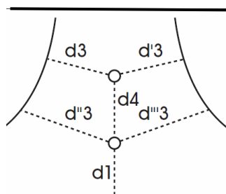
Cas d'une armature par nervure
