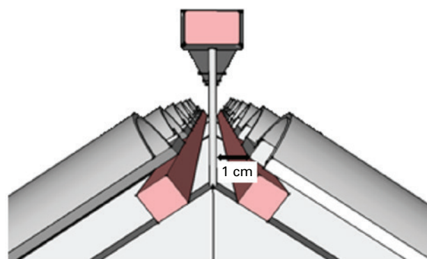
Figure 5 – Dernier liteau au faîtière sans closoir
