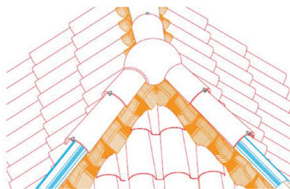
Figure 7 – Jonction de closoirs d'arêtiers et de faîtage dans le cas de tuiles
