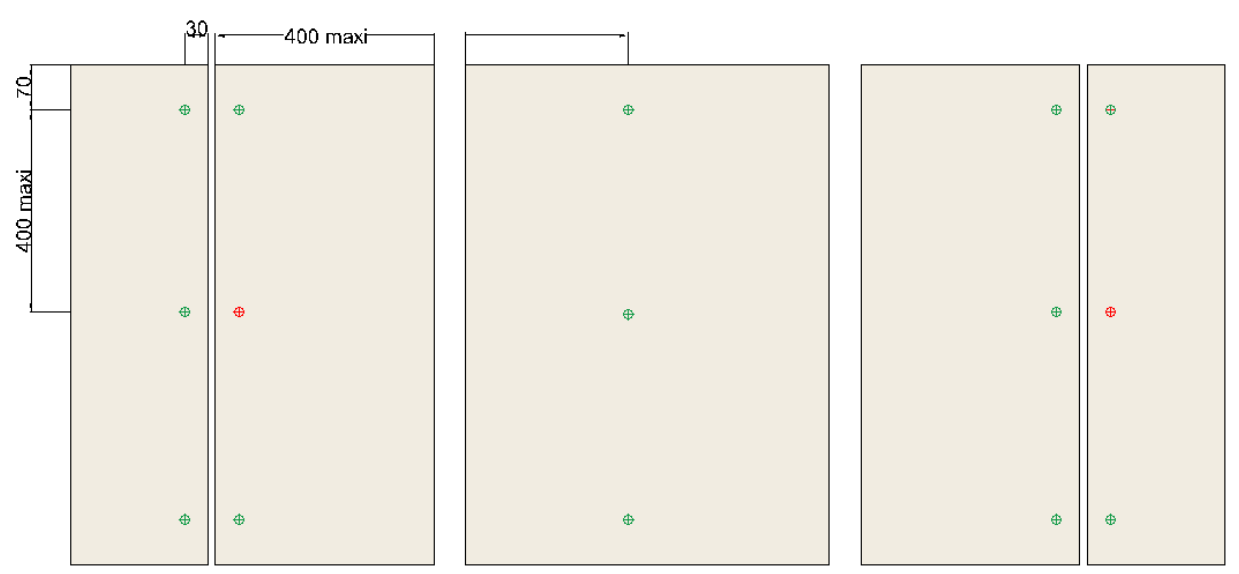
Figure 30 – Pose en sous-face de dalle
