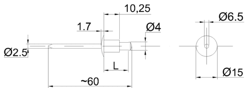
Rivet acier 4x18 K15 A2 (304)
