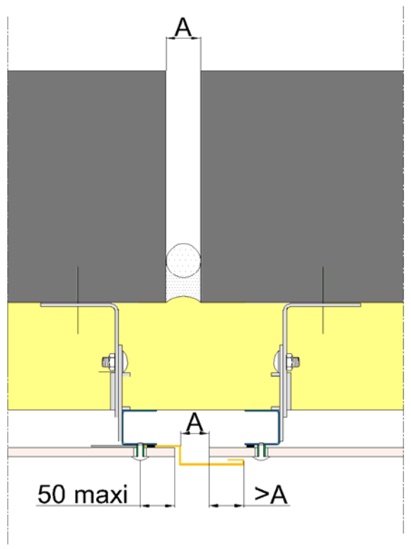
Figure 34 – Joint de dilatation de 12 à 15 cm
